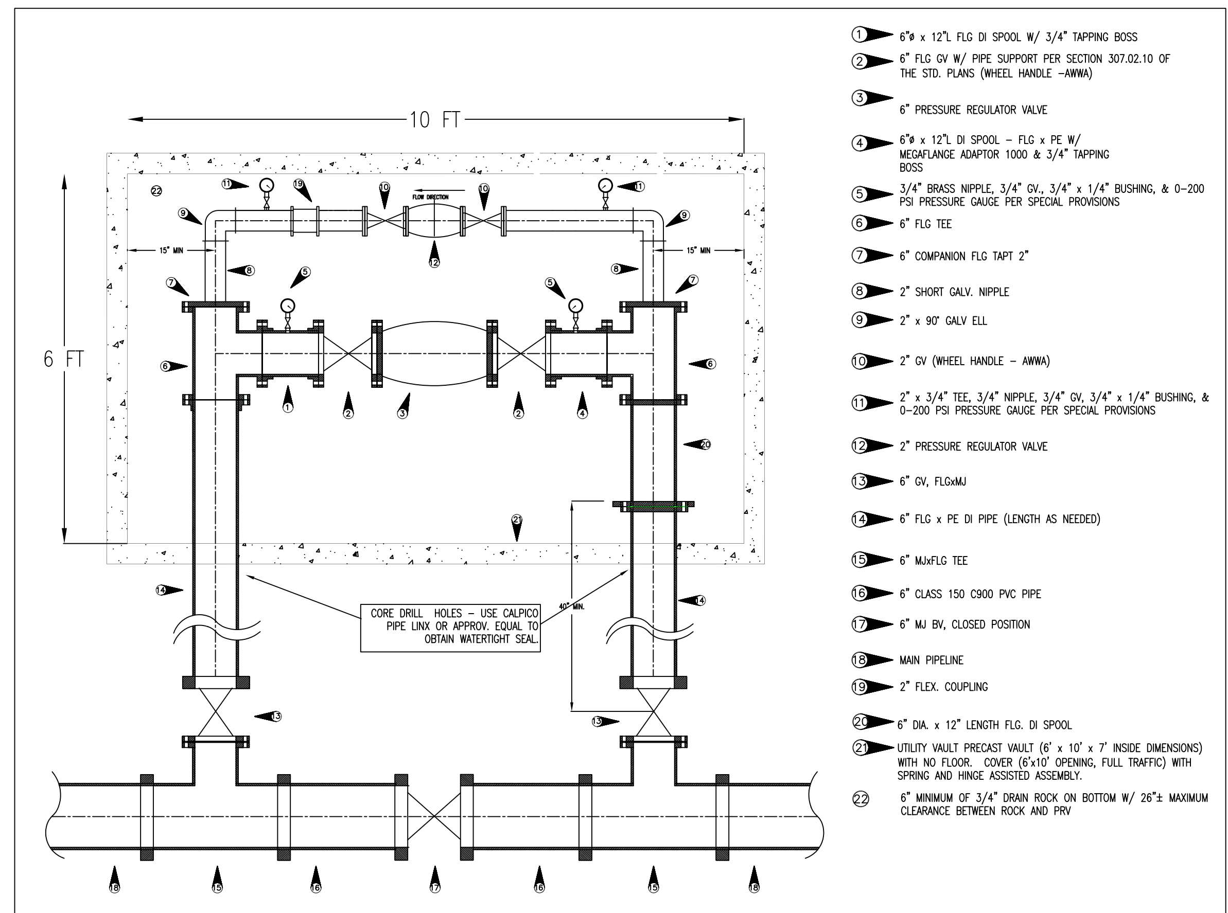
NEW PRV DETAIL N.T.S.
